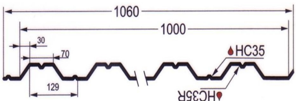
Профнастил GL(Н) 75
