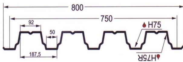
Профнастил GL(Н) 75
