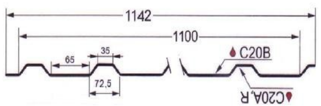
Профнастил GL(НС) 35
