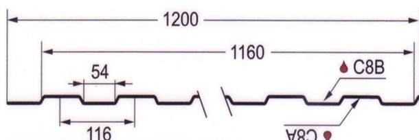
Профнастил GL(C) 10
