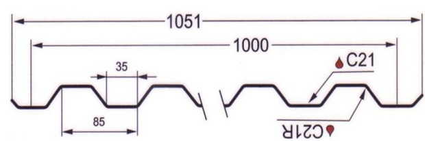
Профнастил GL(Н) 60
